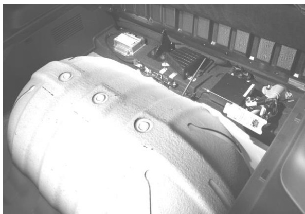
Рисунок 3 – Один из двух баков с водородом, находящихся под днищем автомобиля
