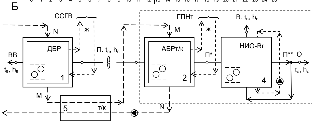
Рисунок 3 – Анализ возможностей солнечной системы кондиционирования воздуха ССКВ; протекающие процессы на H-X диаграмме влажного воздуха (А). Сравнительные возможности ССКВ на основе НИОг (рисунок 1Б) и НИО-Rг (рисунок 3Б). Обозначения в тексте статьи
