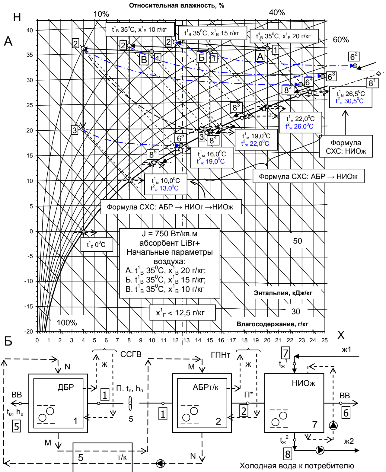
Рисунок 4 – Анализ возможностей солнечной холодильной системы СХС; протекание процессов на Н-Х диаграмме. Принципиальная схема СХС. Влияние влагосодержания наружного воздуха. Обозначения: 1-2 – осушение воздуха; 2-3 – охлаждение основного «О» и вспомогательного «В» воздушных потоков в НАОЖ; 2-6 – изменение состояния воздушного потока в градирне, в соответствии с вариантами работы СХС ( 6^2 - 6^5 ); 8^1 - 8^2 - 8^3 - 8^4 - 8^5 температура охлажденной воды в НАОЖ, в соответствии со схемой СХС, эти точки показаны условно на \varphi = 100\% )
